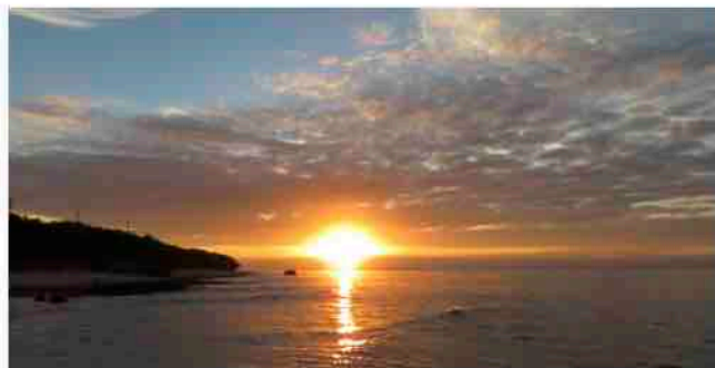
石垣島の朝は遅い 10月31日(土) 6:50 日の出
